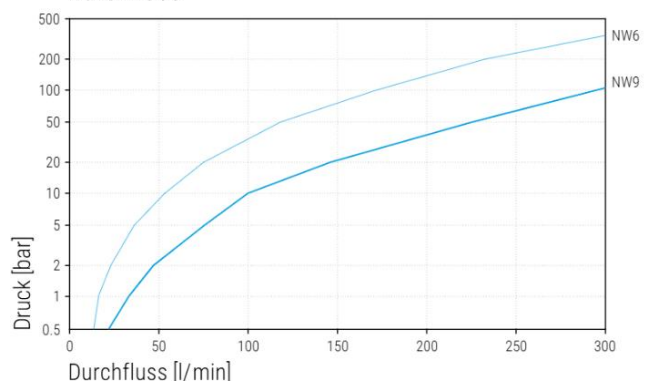
Durchfluss
